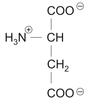
Aspartat
