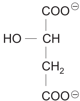
Malat
