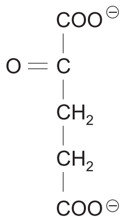
\alpha -Ketoglutarat
