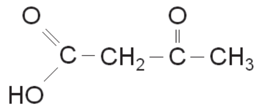
Acetoacetat
