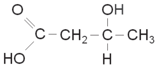
β-Hydroxybuttersäure
