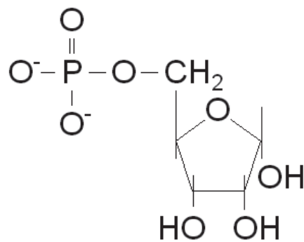
D-Ribose-5-Phosphat
