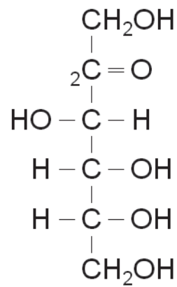
D-Fructose
