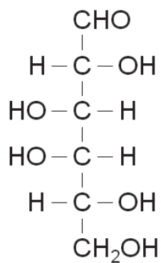
D-Galaktose
