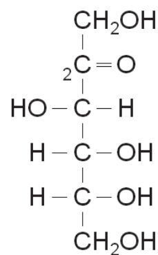
D-Fructose
