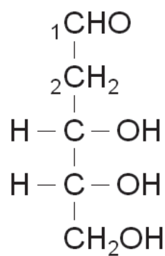
D-Desoxyribose
