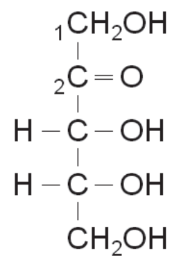
D-Ribulose
