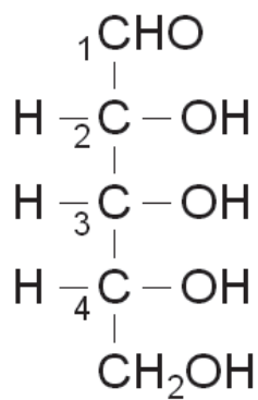
D-Ribose
