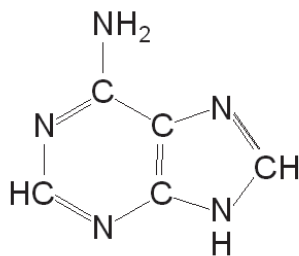
Adenin (Ade)
