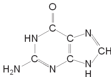
Guanin (Gua)
