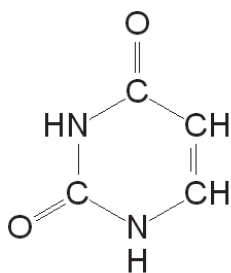
Uracil (Ura)
