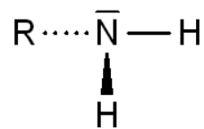
primäres Amin
