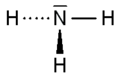
Ammoniak
