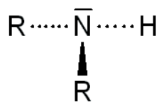
sekundäres Amin
