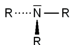
tertiäres Amin
