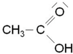
Essigsäure
