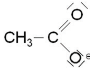
Acetat
