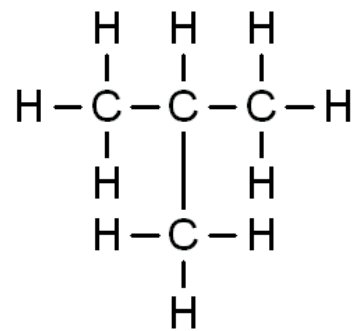
Isobutan
