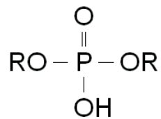
-diester
