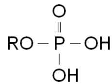
-monoester
