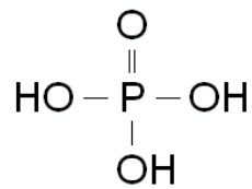
Phosphorsäure
