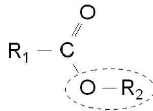
Ester
