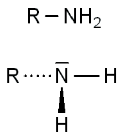
primäres Amin
