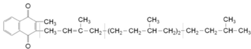
Vitamin K 1 , Phyllochinon (3 Isopreneinheiten)
