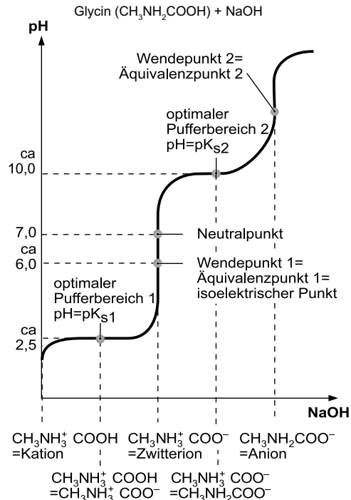
Abb. 19c: Titrationskurve Aminosäure + starke Base
