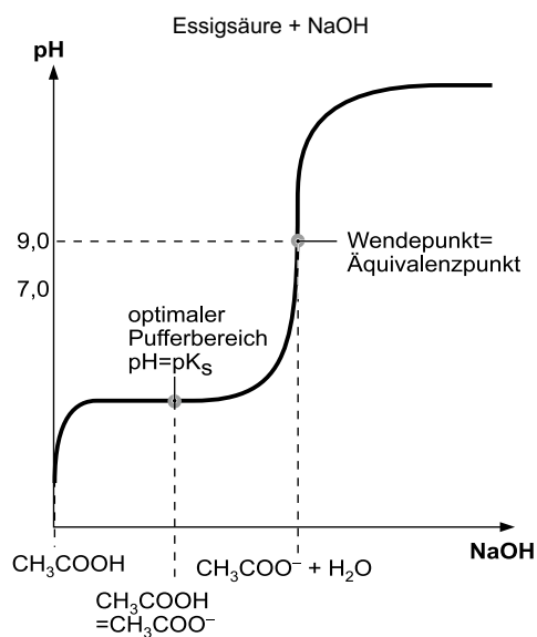
Abb. 19b: Titrationskurve schwache Säure + starke Base
