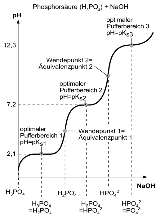
Abb. 19d: Titrationskurve 3-protonige Säure + starke Base
