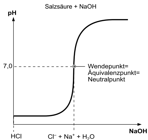
Abb. 19a: Titrationskurve starke Säure + starke Base
