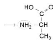
L- Alanin
