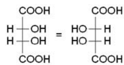
meso - Weinsäure
