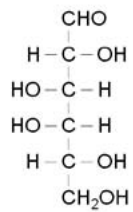
D-Galaktose
