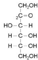
D-Fructose
