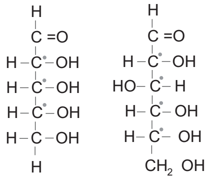
D-Ribose
