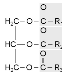
Triglycerid
