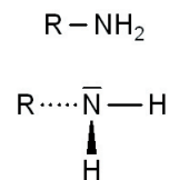
primäres Amin
