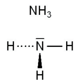
Ammoniak
