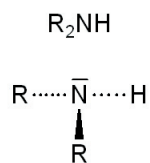
sekundäres Amin
