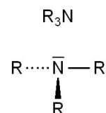
tertiäres Amin
