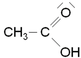
Essigsäure
