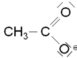
Acetat
