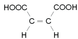
Maleinsäure (Cis-Isomer)
