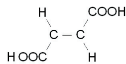
Fumarsäure (Trans-Isomer)
