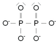
Phosphorsäure- anhydrid
