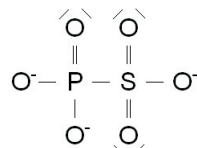
gemischtes Anhydrid
