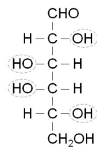
D - Galaktose
