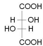
L-(+)-Weinsäure
