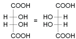
meso - Weinsäure
