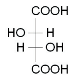
D-(-)-Weinsäure
