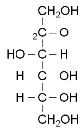
D-Fructose
