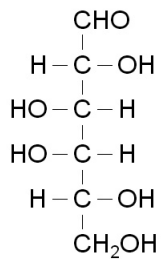
D-Galaktose
