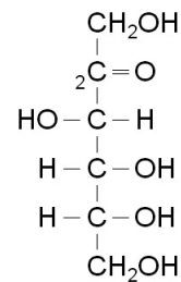
D-Fructose
