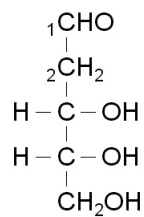
D-Desoxyribose
