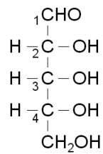
D-Ribose
