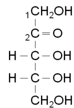
D-Ribulose
