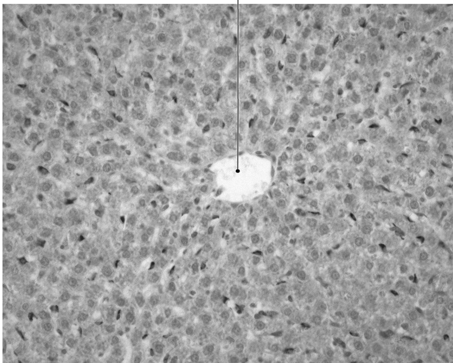
Vena centralis
